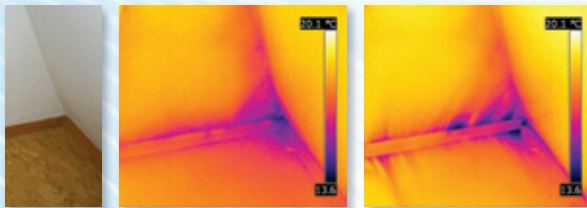
Thermogramm einer Luftleckage
